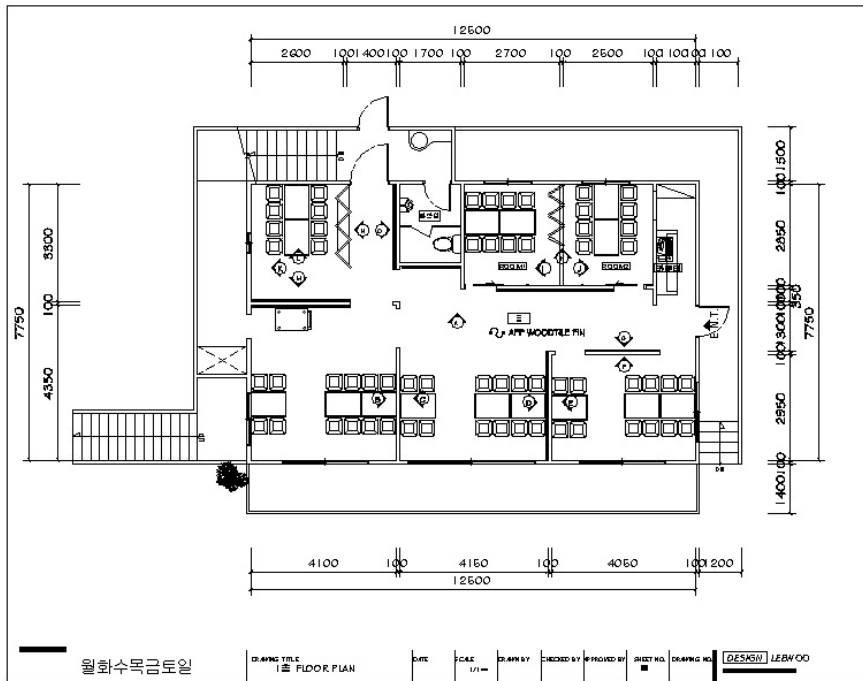
출처: 교육부(2014). 식음료 업장관리(LM1203020301_13v1). 한국직업능력개발원. p.4. [그림 1-1] 식음료 업장 설계도
